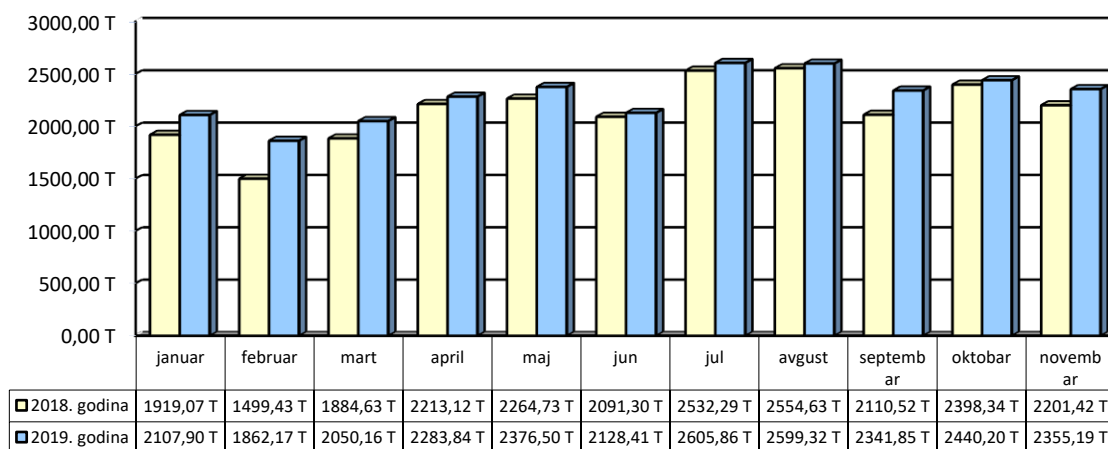
Grafikon 3 - Količine deponovanog otpada u 2018. i 2019. godini
